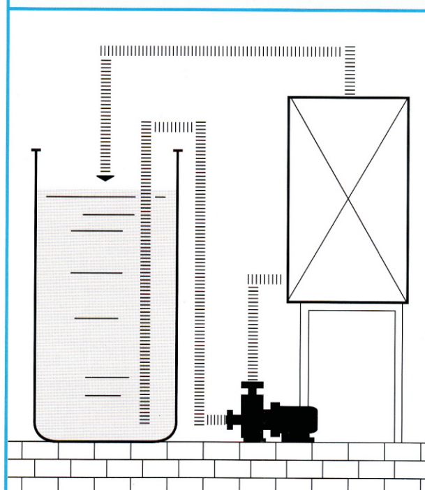
两缸液体之热循环， 过滤及混合
