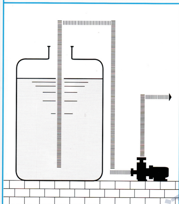
从大型水箱液面吸出及输送
