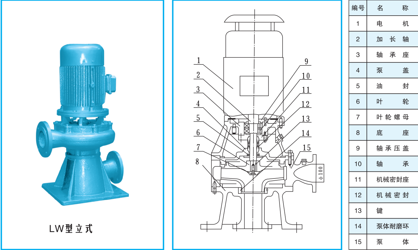
<<< LW型泵安装外型图 >>>
