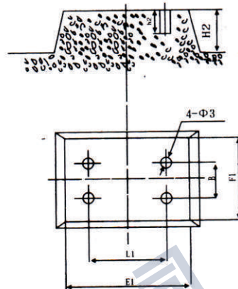
(二)、硬性联接基础图
