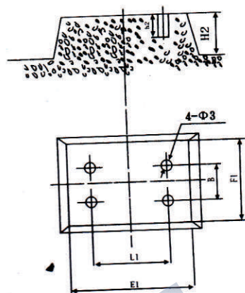
(二)、硬性联接基础图
