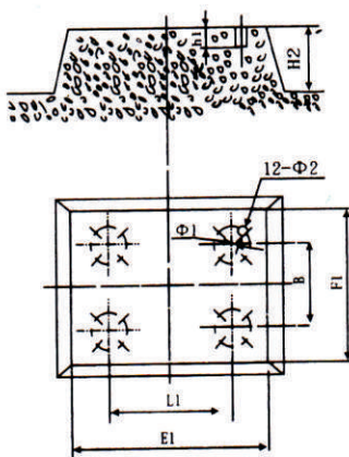
(一)、柔性联接基础图
