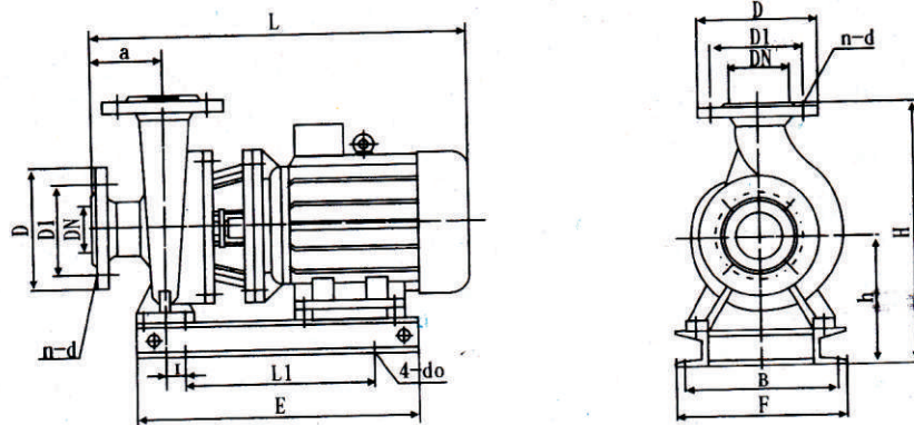
<< ISWD、ISWRD、ISWHD、ISWYD、ISWHYD型系列泵安装尺寸图表 >>
