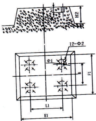
(一)、柔性联接基础图
