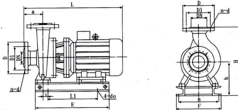
<< ISW、ISWR、ISWH、ISWY、ISWHY型系列泵安装尺寸图表 >>
