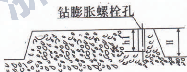
(一)、柔性联接基础图
