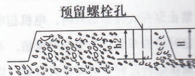
(二)、硬性联接基础图
